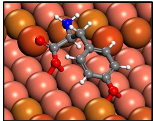
L-Tyr
