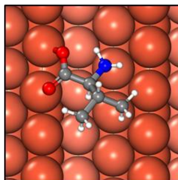
Val-(211)
