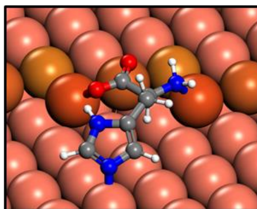
L-His
