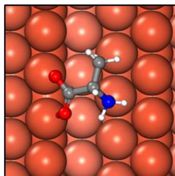
Ala-(211)
