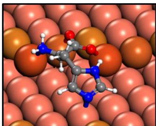
D-His
