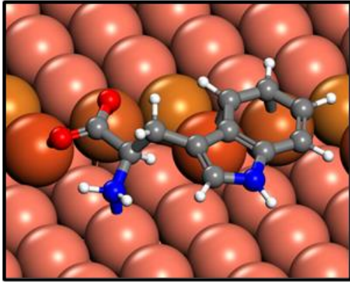
D-Trp
