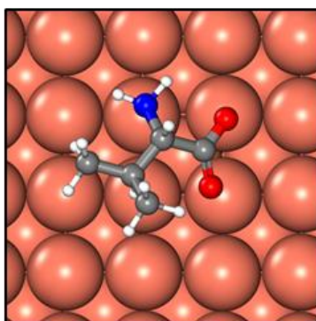
Val-(100)
