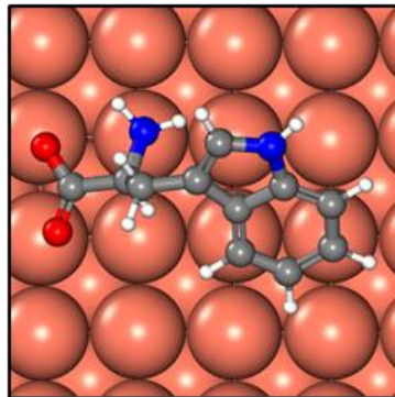
Trp-(100)
