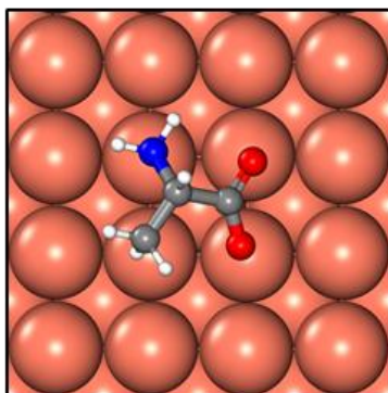
Ala-(100)
