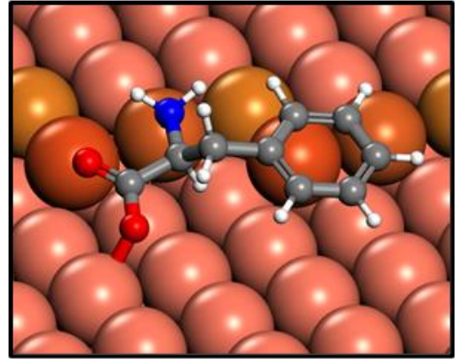
L-Phe
