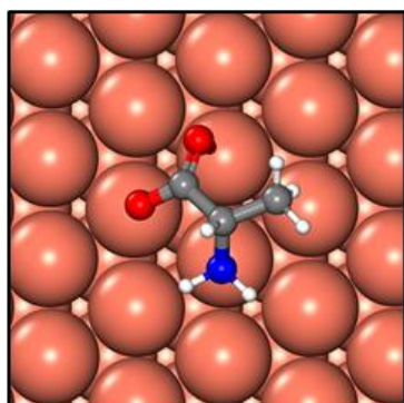
Ala-(111)
