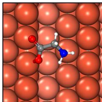
Gly-(211)
