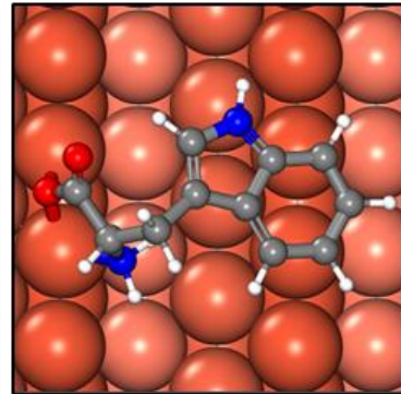
Trp-(211)
