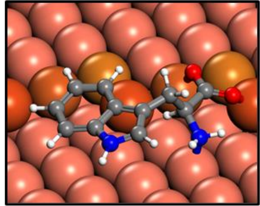
L-Trp
